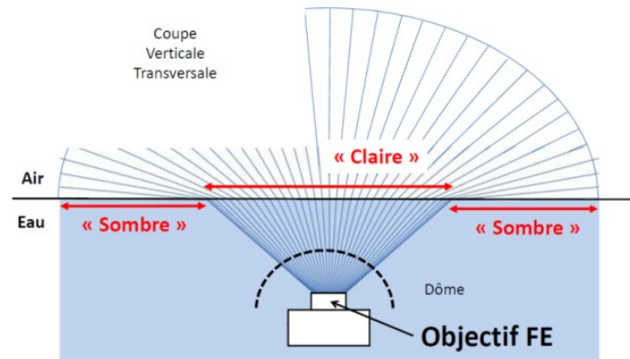
Fenêtre de Snell
